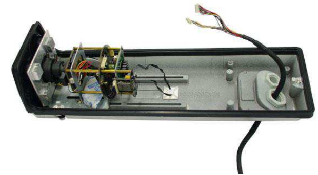
5-2. 글랜드를 통해 외부에서 내부로 케이블을 삽입하고 단자대를 다시 연결 합니다.
