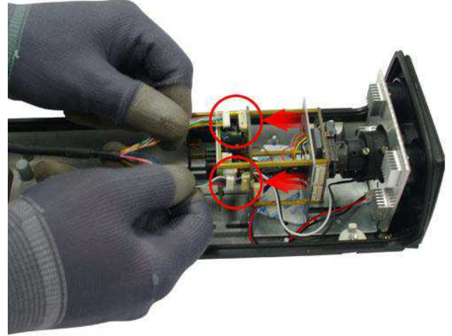
4. 2개의 단자대를 제거 합니다.
