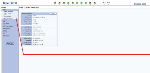
<소프트웨어 화면 >
