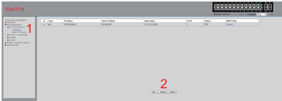
<소프트웨어 화면 >
