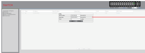
<소프트웨어 화면 >
